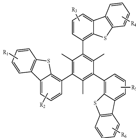
Compound 6G
