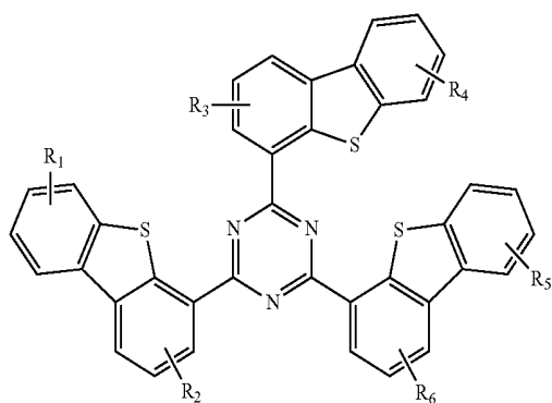
Compound 6G
