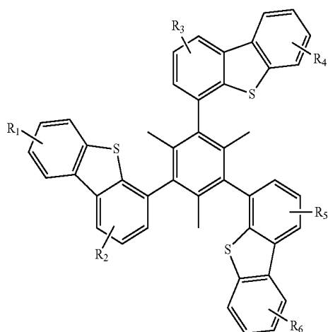
Compound 6G
